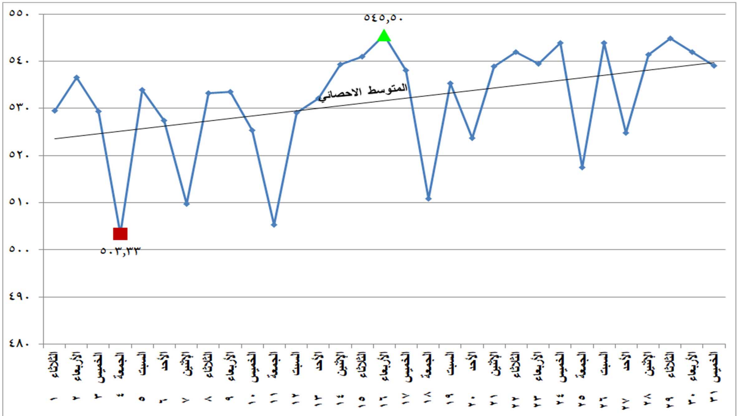
شكل (١٥) إجمالي الطاقة الكهربائية المنتجة من كل المصادر الأولية خلال شهر مارس ٢٠٢٢
