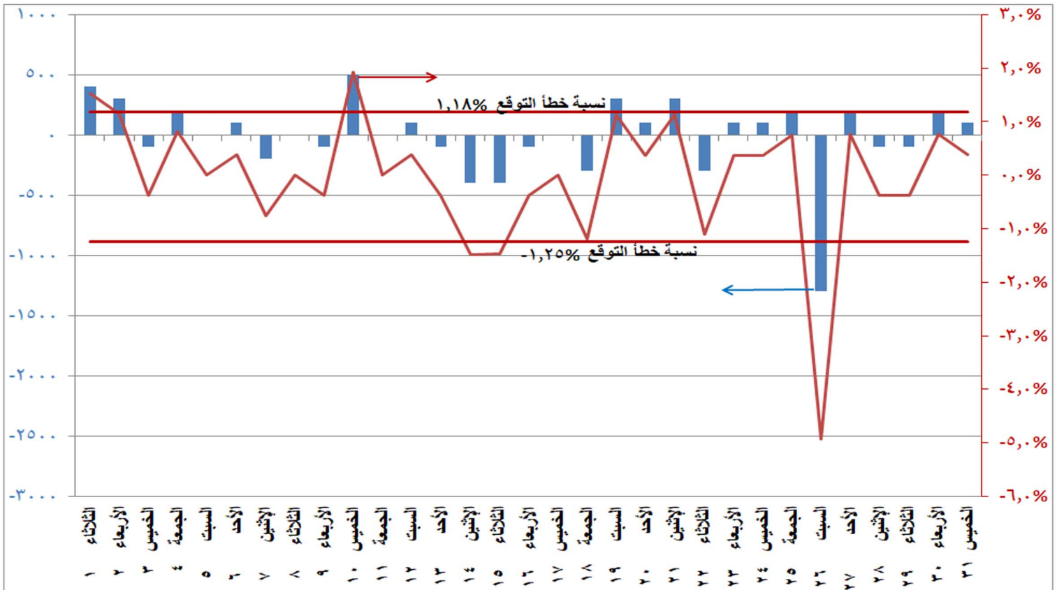
شكل (١٠) الفرق بين الحمل الأقصى المتوقع والمسجل فعليا ونسبة الفرق إلى الحمل المسجل فعليا خلال شهر مارس ٢٠٢٢
