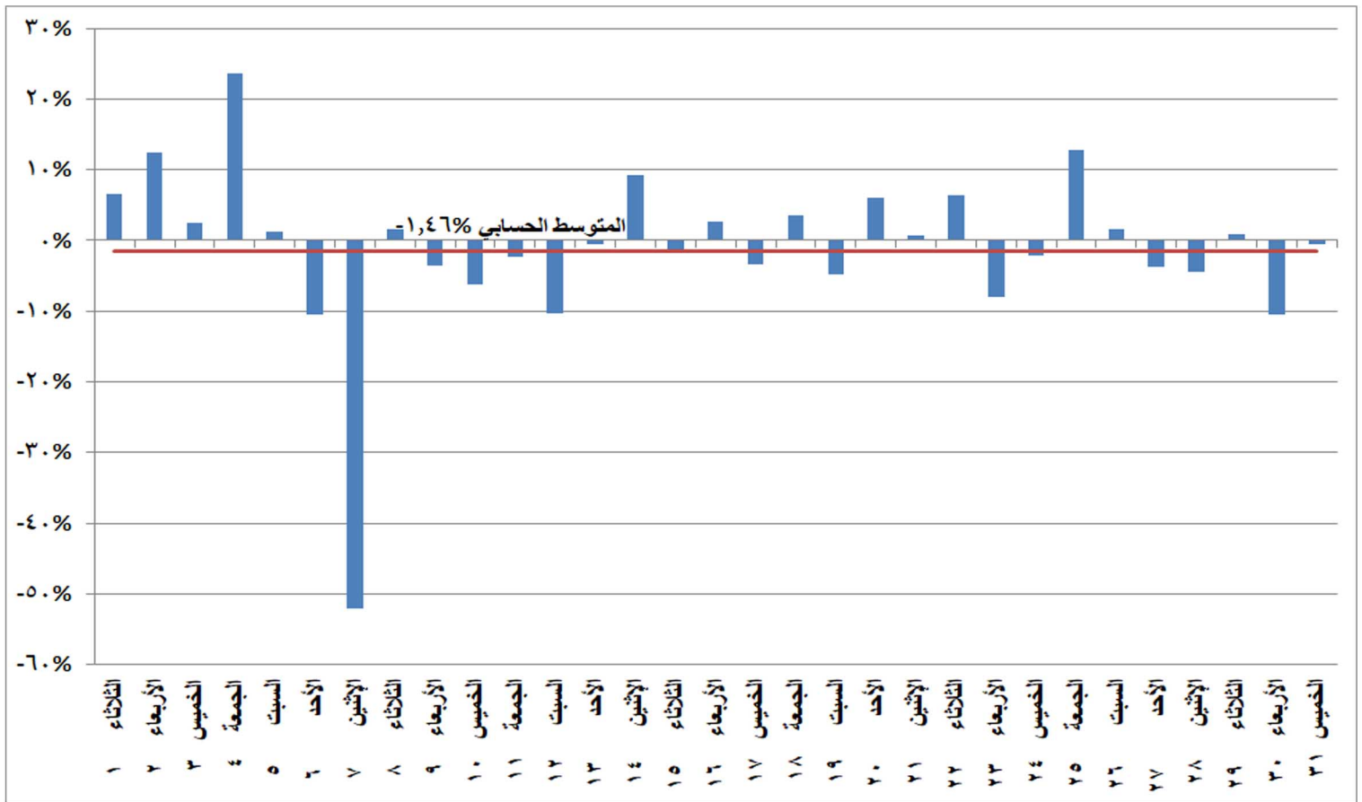
شكل (٢٤) نسب التغير في استخدام المصادر المائية في إنتاج الطاقة الكهربائية خلال شهر مارس ٢٠٢٢ مقارنة بالشهر المماثل من العام السابق
