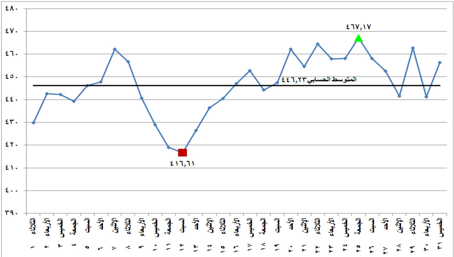
شكل (١٤) معامل انبعاثات غاز ثاني اكسيد الكربون المكافئ على مدى شهر مارس ٢٠٢٢
