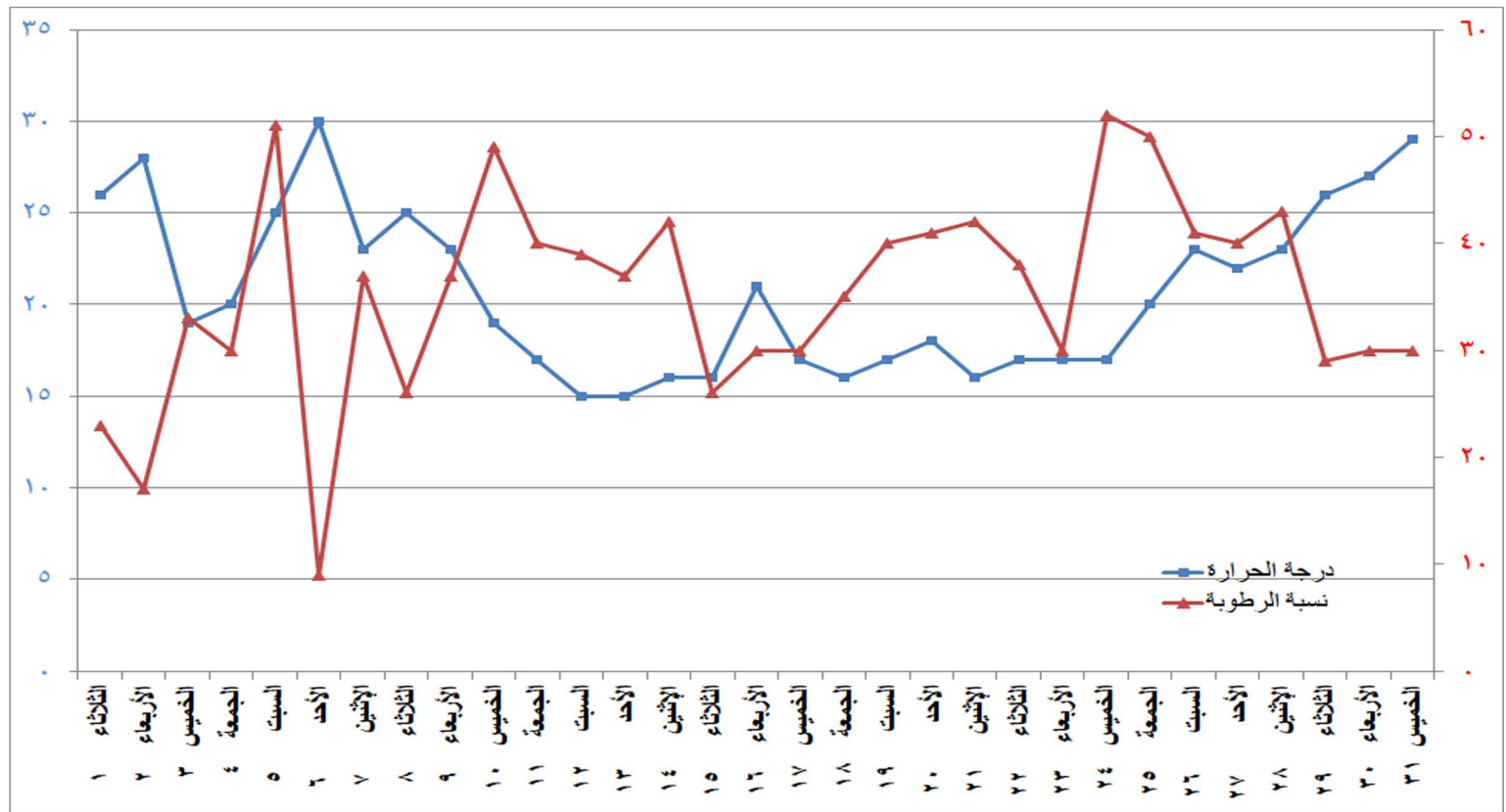
شكل (١١) التغيير في درجة الحرارة والرطوبة النسبية خلال شهر مارس ٢٠٢٢
