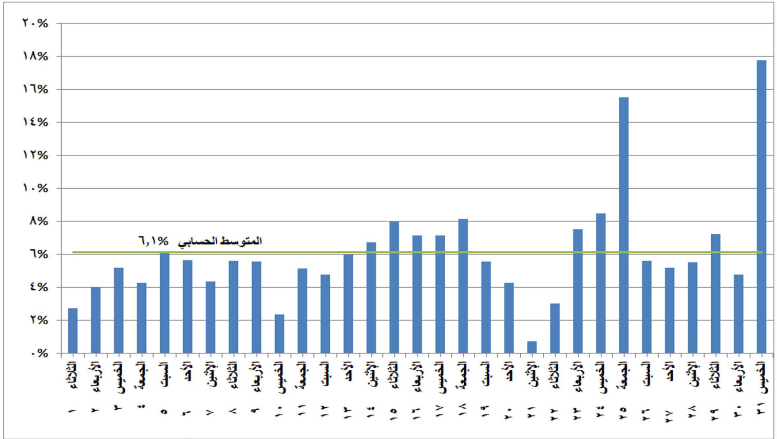
شكل (٩) النسب المئوية للتغير في الحمل الاقصى خلال شهر مارس ٢٠٢٢ مقارنة باليوم المماثل من العام الماضي
