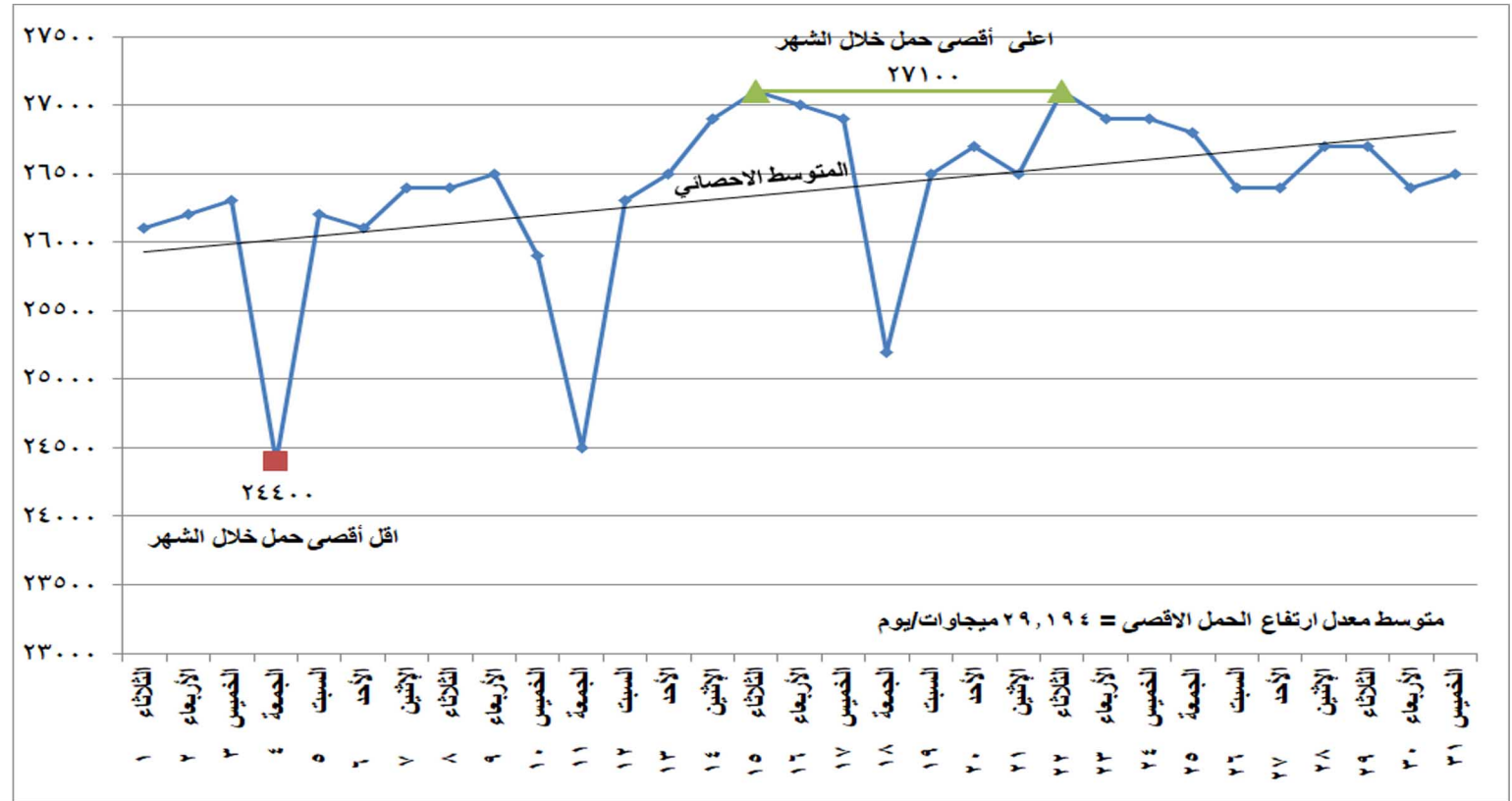
شكل (١) تطور الحمل الاقصى اليومي خلال شهر مارس ٢٠٢٢
