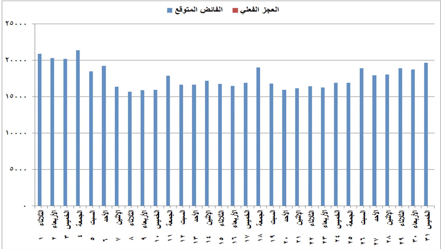
شكل (٧) الفائض والعجز المتوقع للقدرات خلال شهر مارس ٢٠٢٢
