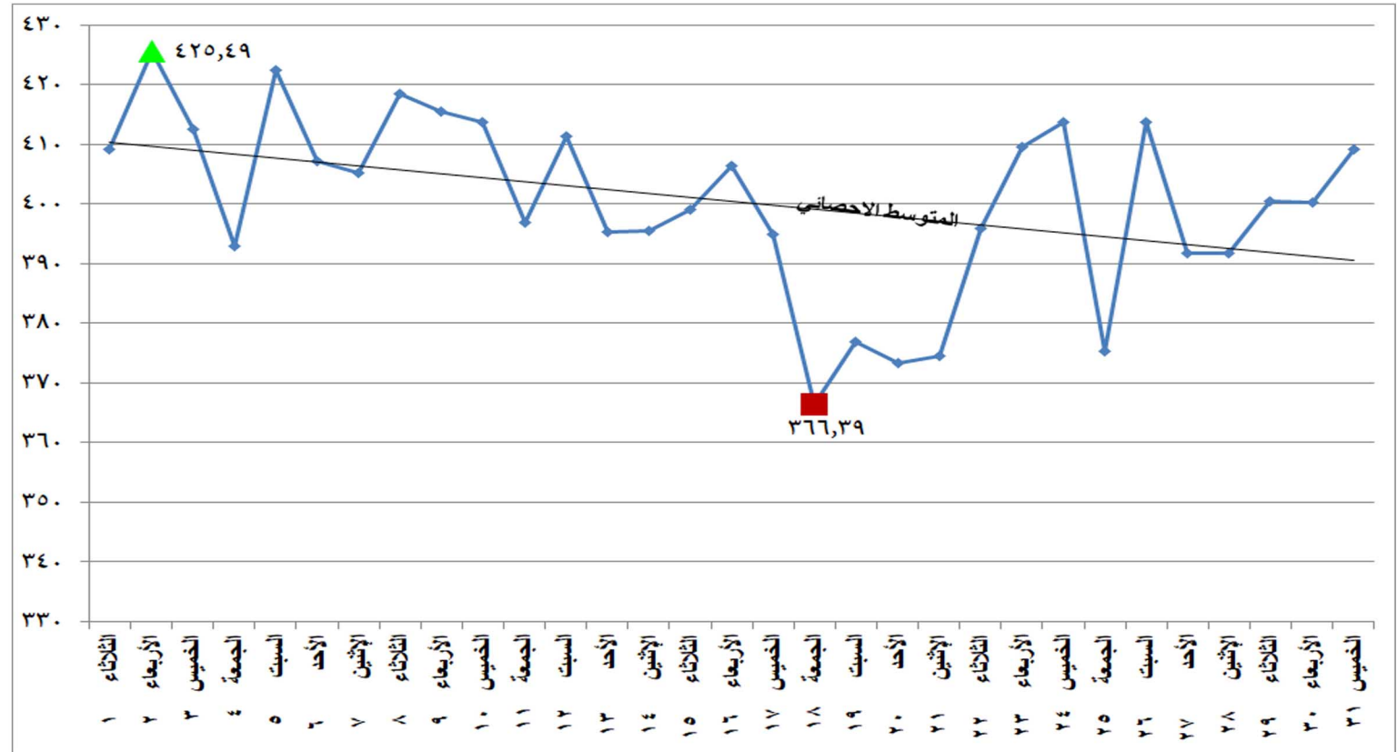
شكل (١٧) الطاقة الكهربائية المنتجة من الغاز الطبيعي خلال شهر مارس ٢٠٢٢
