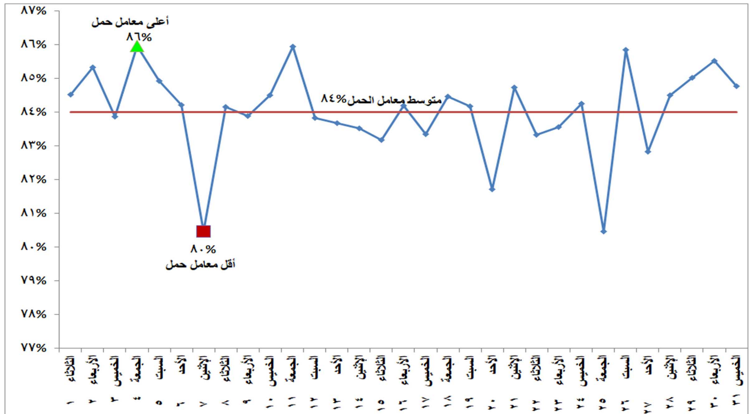
شكل (١٢) إجمالي معامل الحمل لوحدات الانتاج خلال شهر مارس ٢٠٢٢
