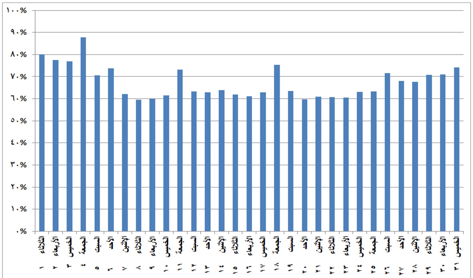
شكل (٢٨) نسب الفائض للحمل الاقصى المسجل يوميا خلال شهر مارس ٢٠٢٢
