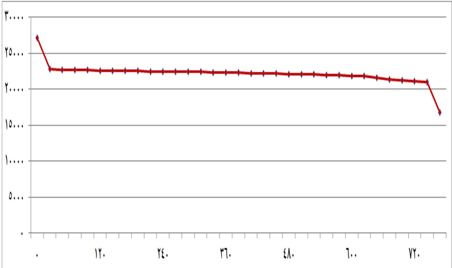
شكل (٧) الفائض والعجز المتوقع للقدرات خلال شهر مارس ٢٠٢٢
