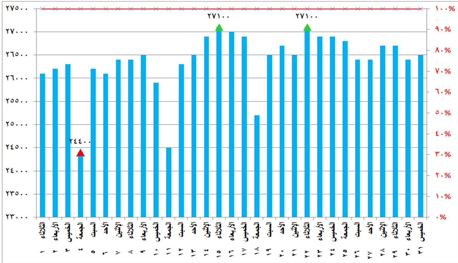
شكل (٥) قدرات الانتاج المتاحة ونسبتها للحمل الاقصى خلال شهر مارس ٢٠٢٢
